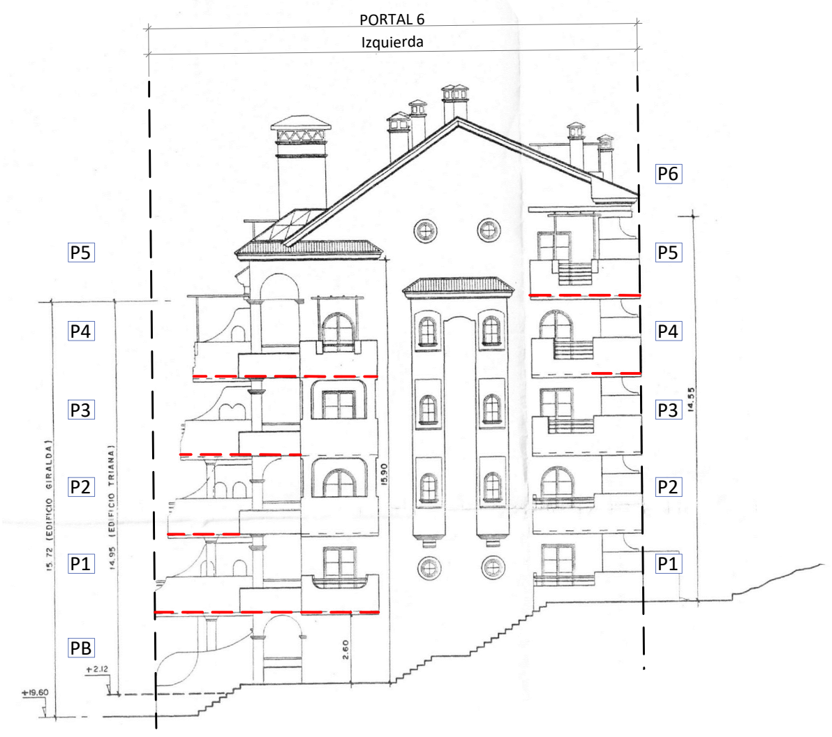
ALZADO LATERAL NOROESTE
